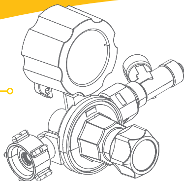
Détendeur Réf. 693
